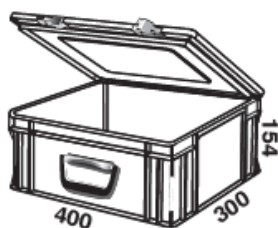
PH-710 ESD Hordozóláda
